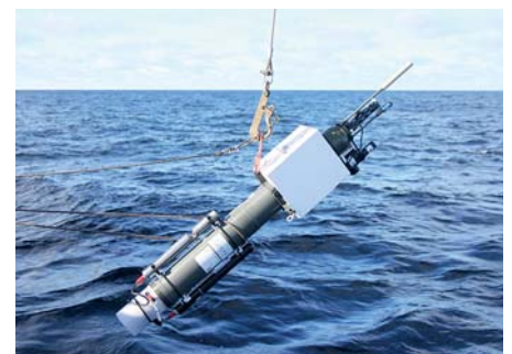
Bestückt mit neuartigen Sensoren für die Nitrat-Messung: Agro-Float vor dem Einsatz. Foto: M. Naumann, IOW
