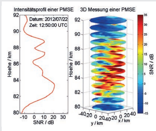
Abb. 3: Herkömmliche Beobachtungsverfahren liefern meist nur ein vertikales Profil durch die PMSE (links). MAARSY ermöglicht es, die dreidimensionale Struktur einer PMSE zu beobachten (rechts).
