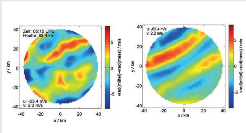
Abb. 4: Die gemessenen radialen Dopplerverschiebungen beinhalten Beiträge verschiedener Wellen. Links: Aus den MAARSY-Messungen lassen sich einzelne Schwerewellen herausfiltern und ihre Eigenschaften bestimmen. Rechts: Diese Eigenschaften werden mit Hilfe von Simulationen überprüft. Grafiken: Gunter Stober, IAP
