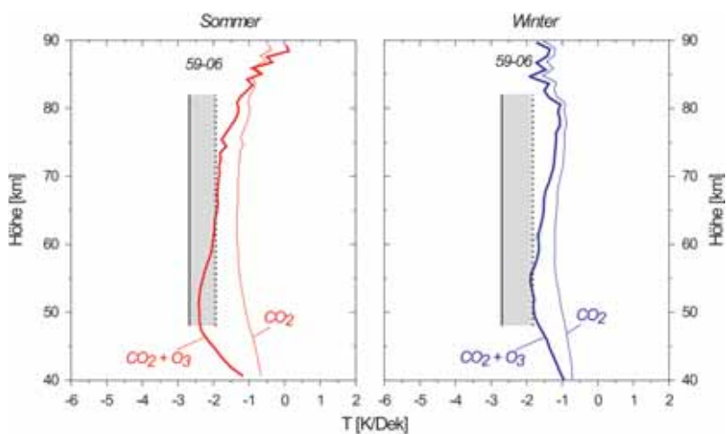
Abb. 2: Mittlere Temperaturtrends aus Feldstärkemessungen (graue Balken) und nach Modellrechnungen für realistische Trends von \text{CO}_2 und Ozon (rote und blaue Kurven), jeweils für Sommer- und Winterbedingungen.
